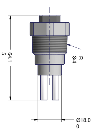
ECDI/0,2
